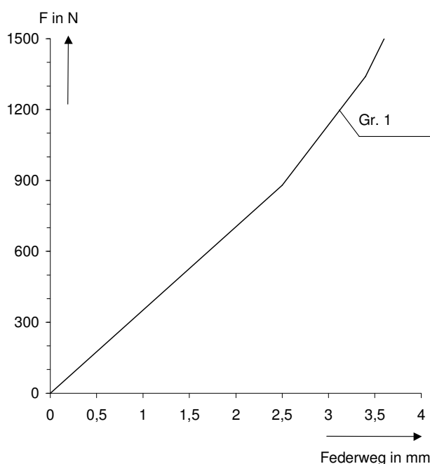
Federkennlinie Gr. 1, 2, 3
