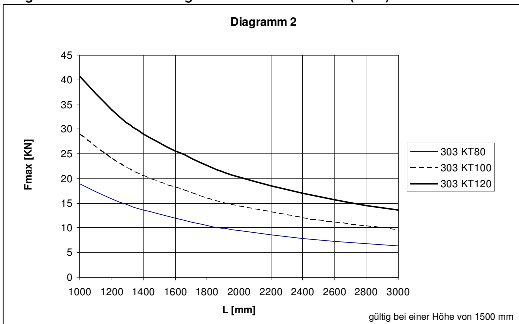
Diagramm 2 : Punktbelastung für freistehende Brücke (Mitte) bei statischer Last
