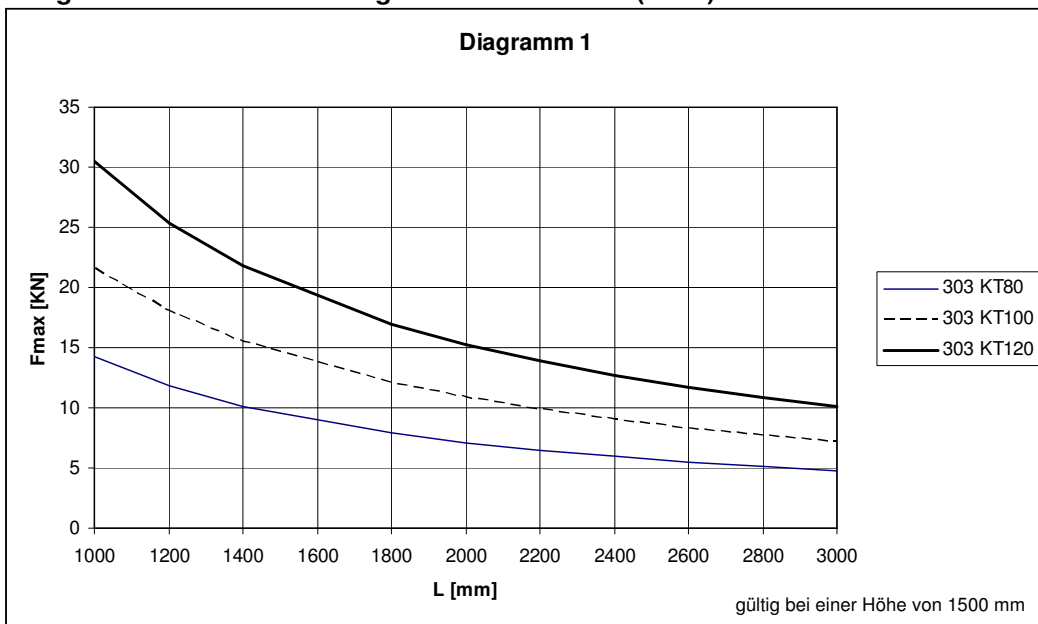
Diagramm 1 : Punktbelastung für Winkelkonsole (Mitte) bei statischer Last
