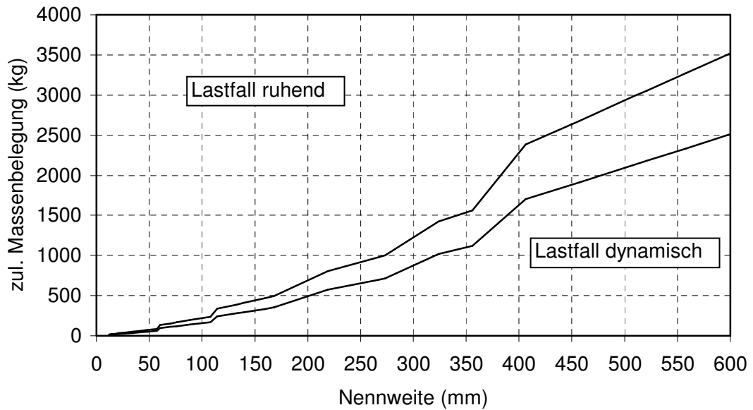
Zul. Massenbelegung für dipa Typ 170 (2 Punkt Aufhängung)
